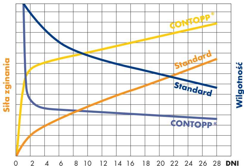
Rysunek 1: linie żółte: wytrzymałość na ściskanie/zginanie linie niebieskie: wilgotność resztkowa.
